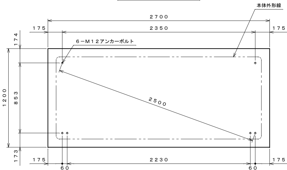
基礎伏せ図 S=1:20
