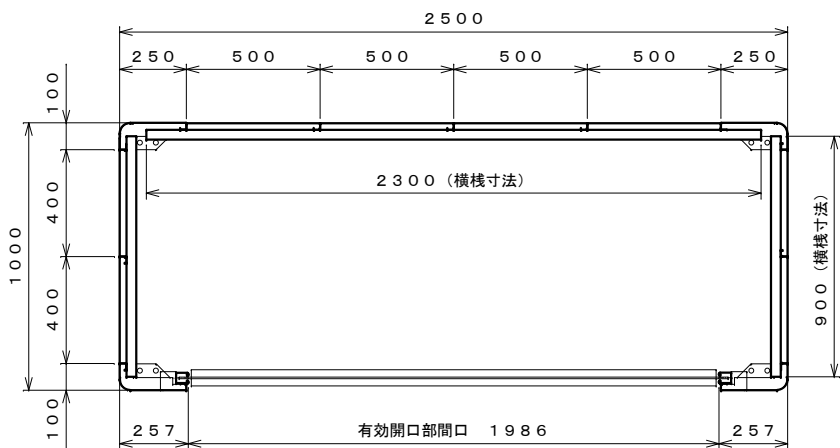
平面図 S=1:20
