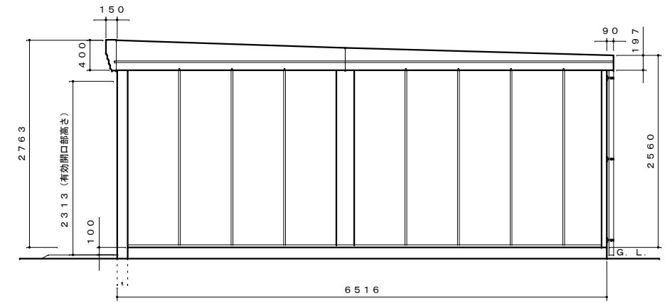
側面図 S=1:50
