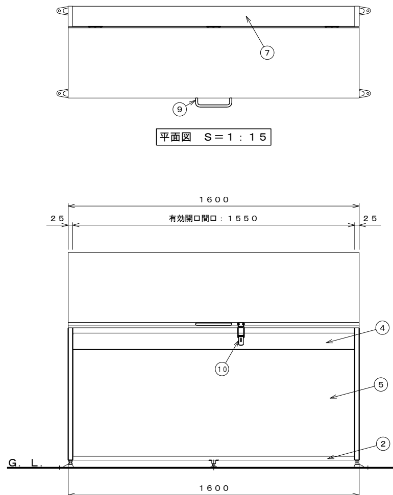
正面図 S=1:15
