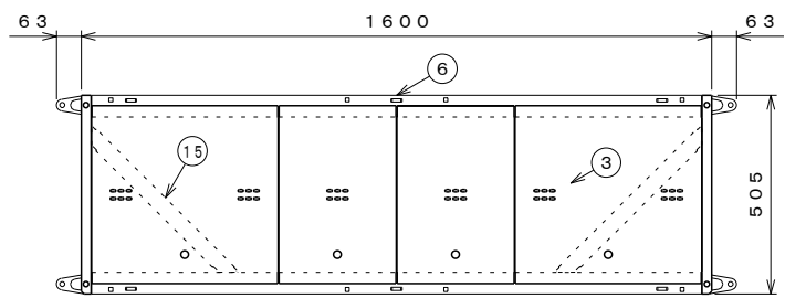
平面断面図 S=1:15
