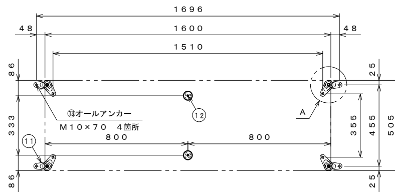
アンカー位置図 S=1:15
