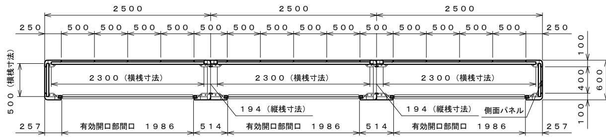
平面図 S=1:40
