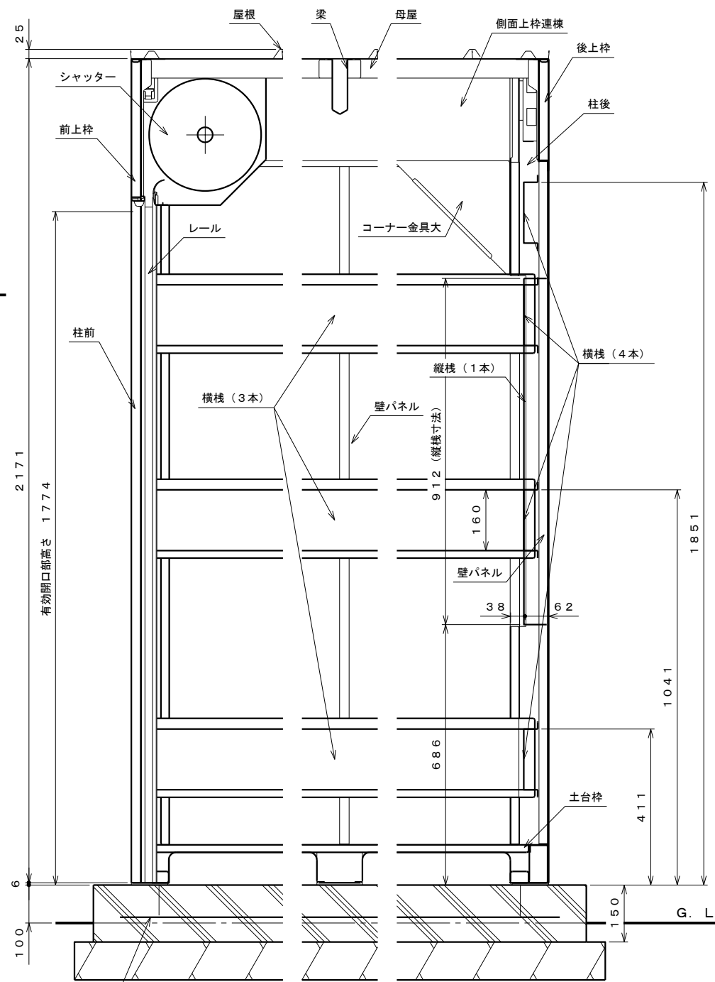
側面断面図 S=1:10
