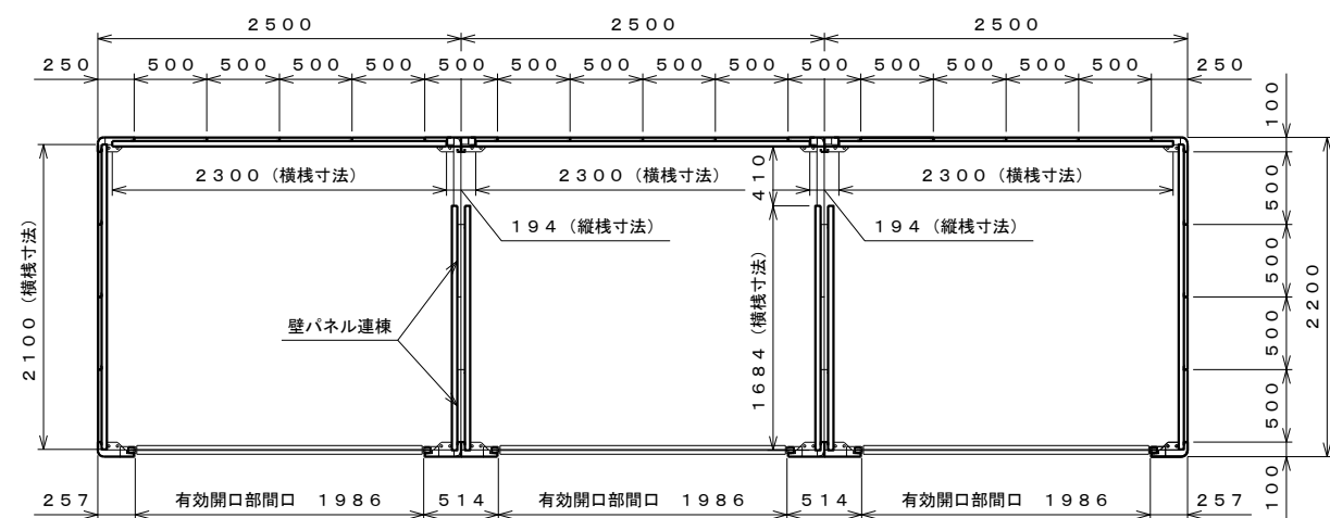
平面図 S=1:40
