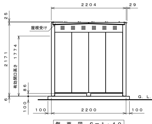
側面図 S=1:40
