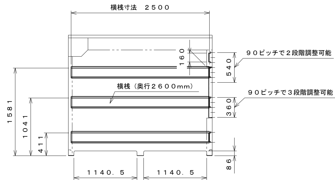
内面図 S=1:40
