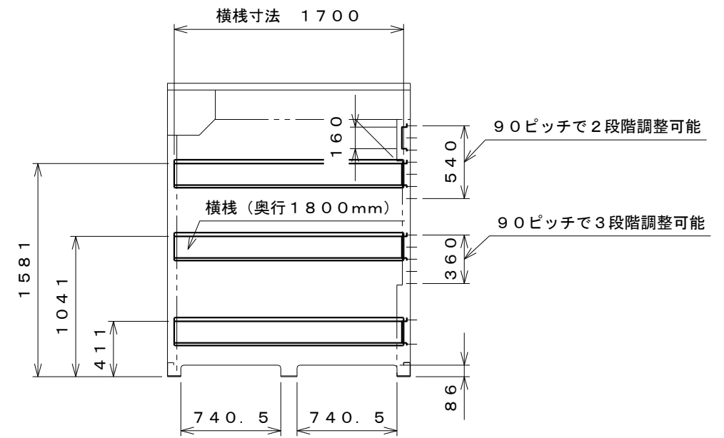
内面図 S=1:40
