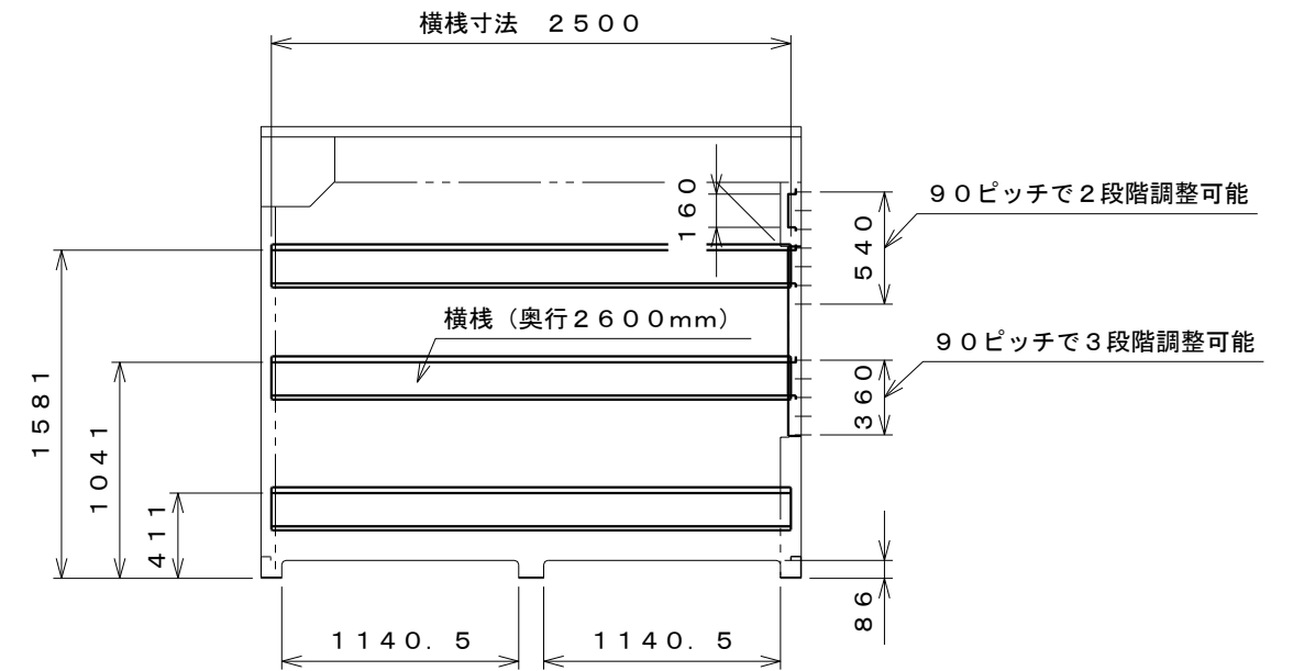
内面図 S=1:40
