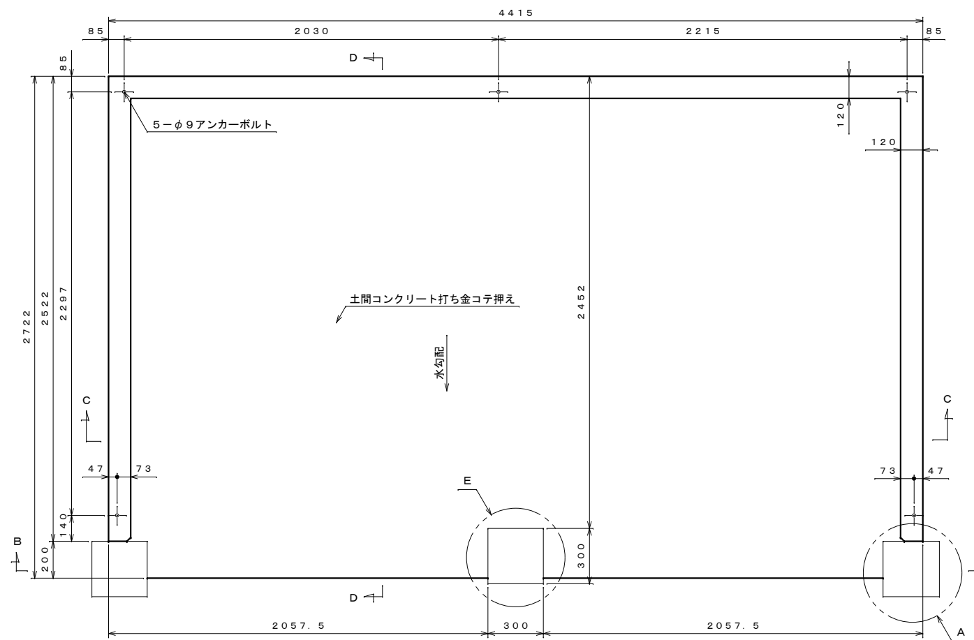
基礎伏せ図 S=1:20
