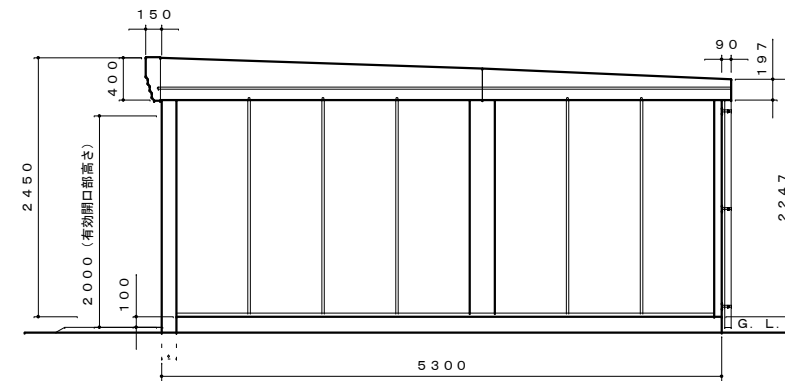
側面図 S=1:50
