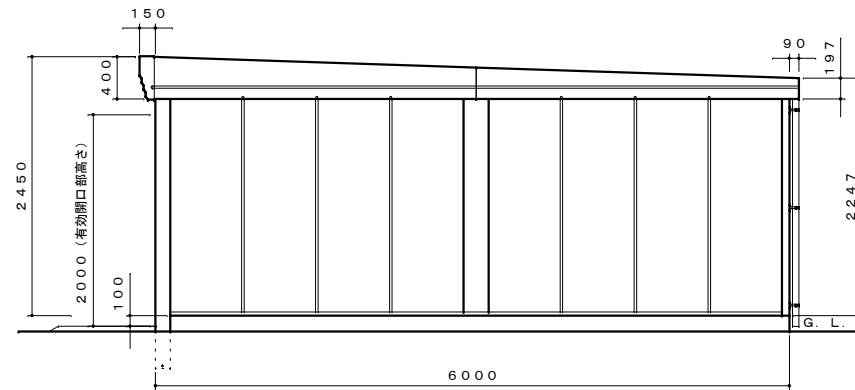
側面図 S=1:50
