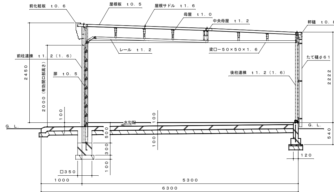
側面断面図 S=1:40
