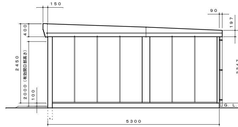
側面図 S=1:50
