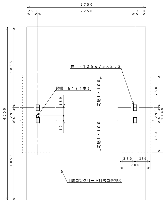
基礎伏せ図 S = 1 : 30
