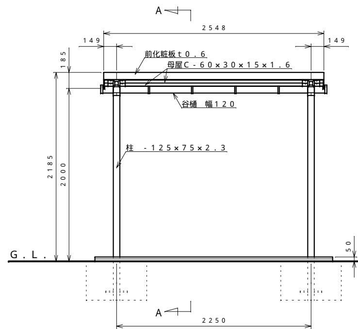
正面図 S = 1 : 30
