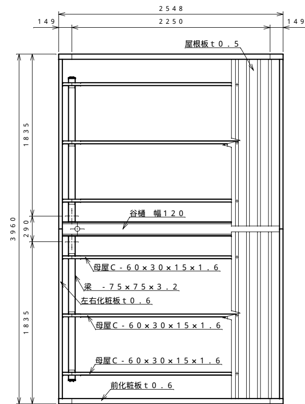
平面図 S = 1 : 30
