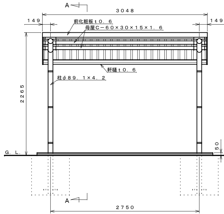
正面図 S=1:30
