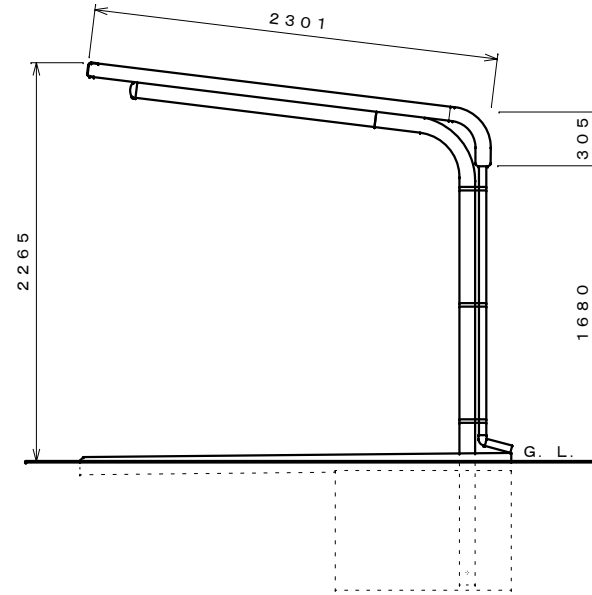
側面図 S=1:30
