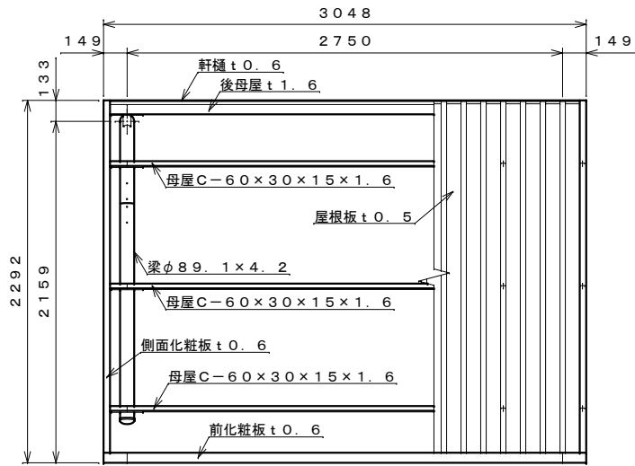
平面図 S=1:30
