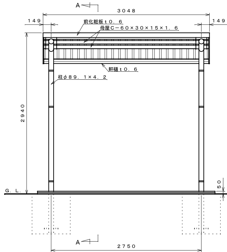
正面図 S=1:30
