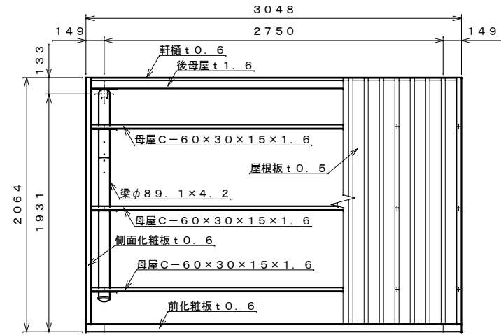
平面図 S=1:30
