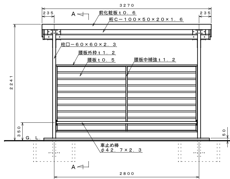
正面図 S=1:30
