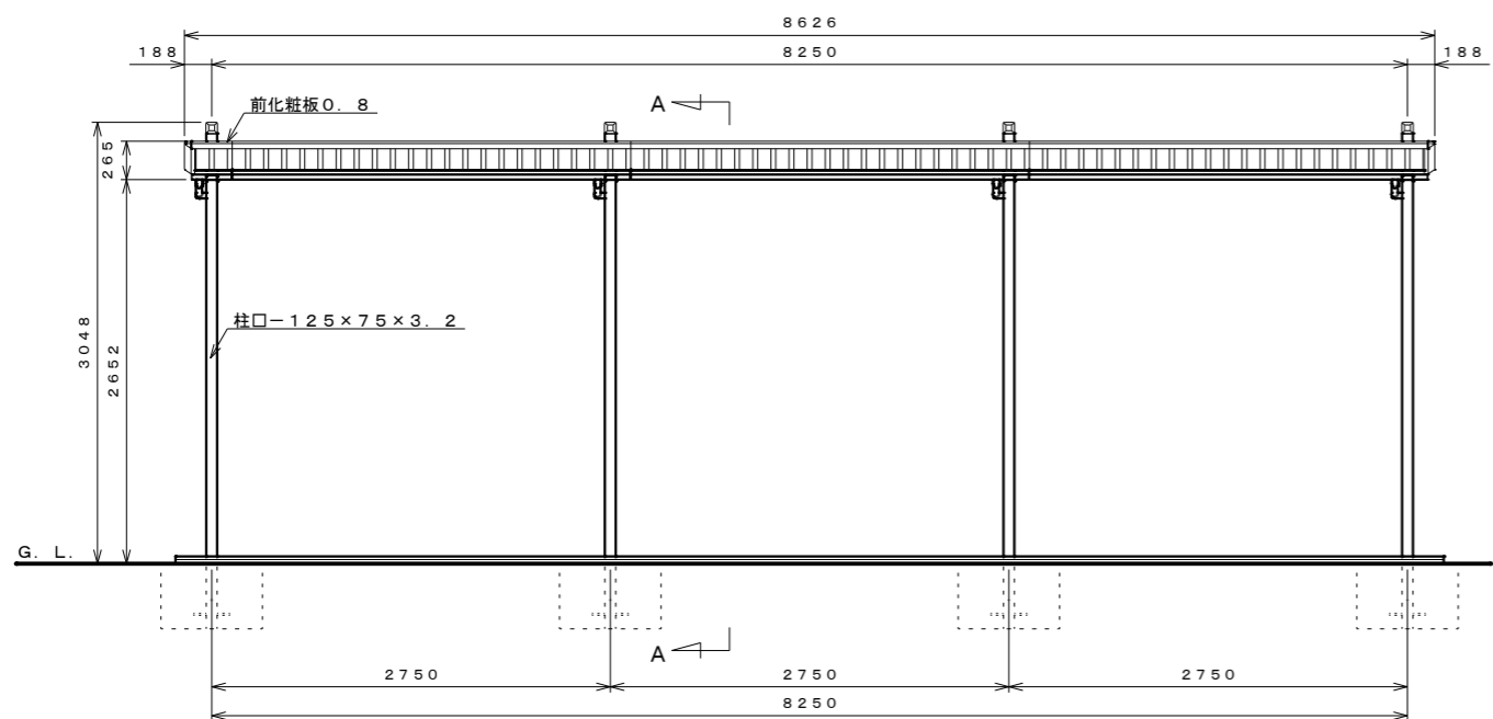
正面図 S=1:40
