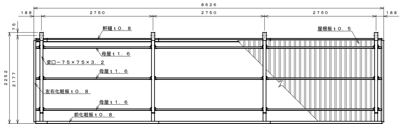
平面図 S=1:40
