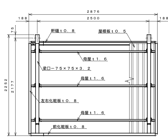
平面図 S=1:30
