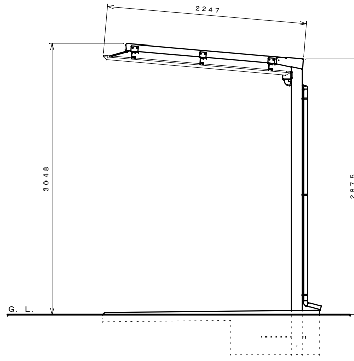
側面図 S=1:30
