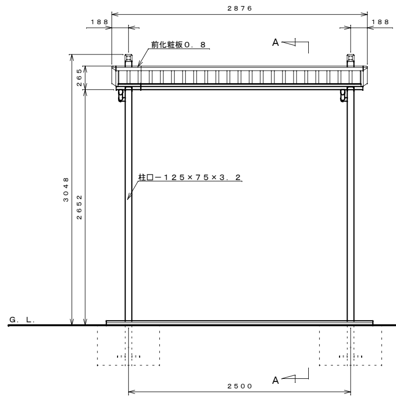
正面図 S=1:30
