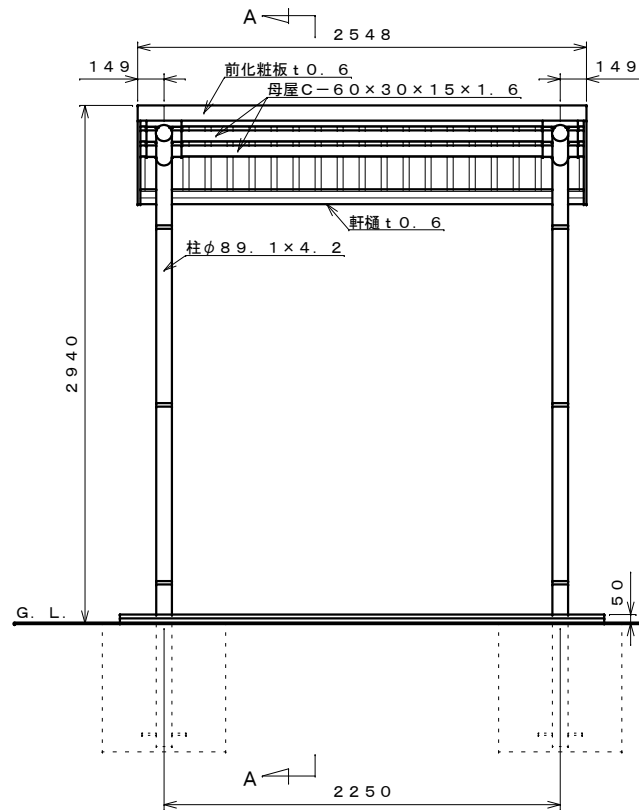
正面図 S=1:30
