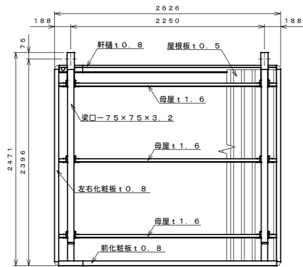
平面図 S=1:30
