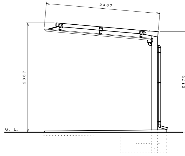
側面図 S=1:30
