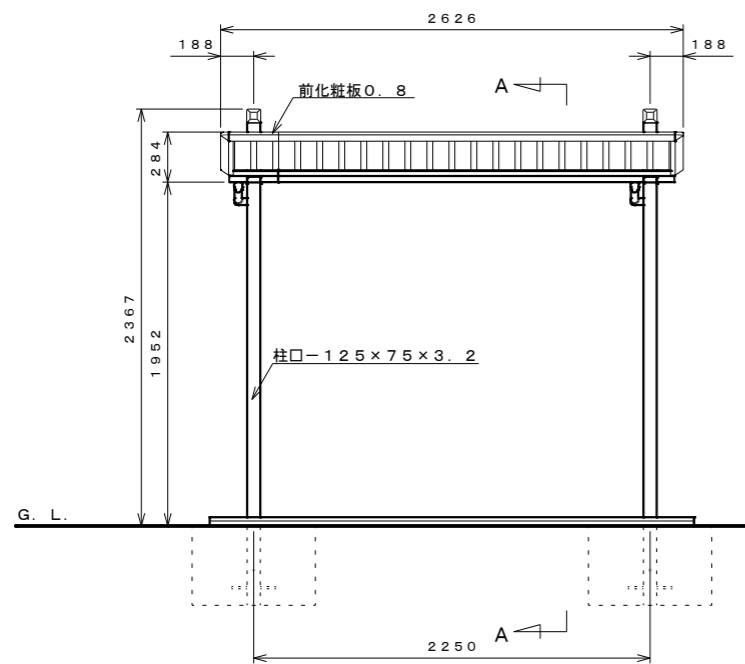
正面図 S=1:30
