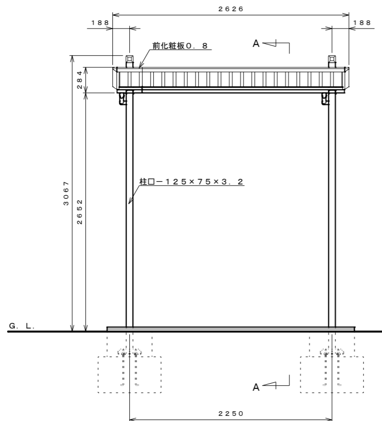
正面図 S=1:30
