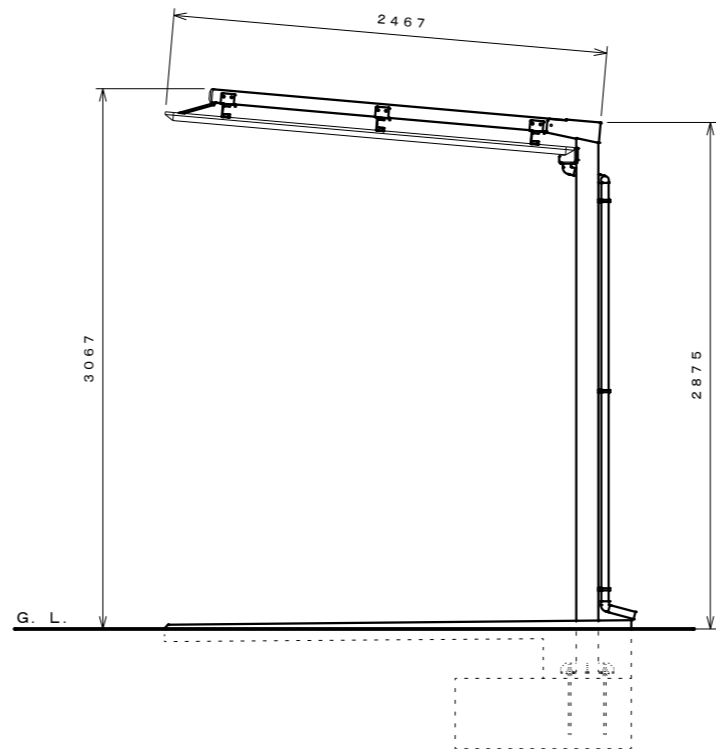
側面図 S=1:30
