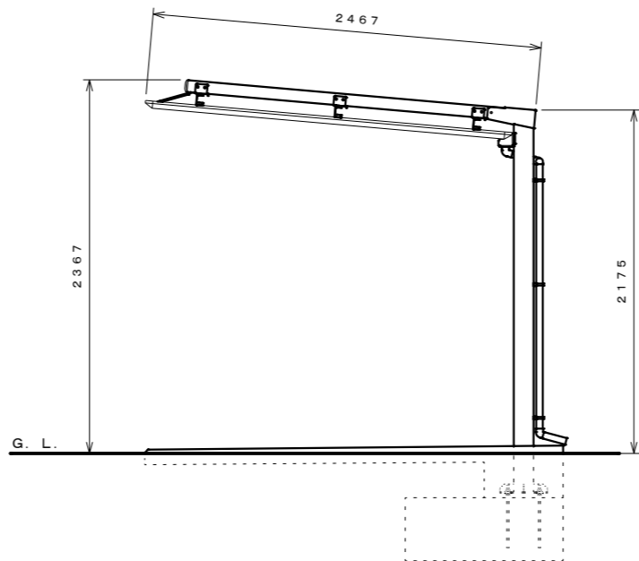
側面図 S=1:30
