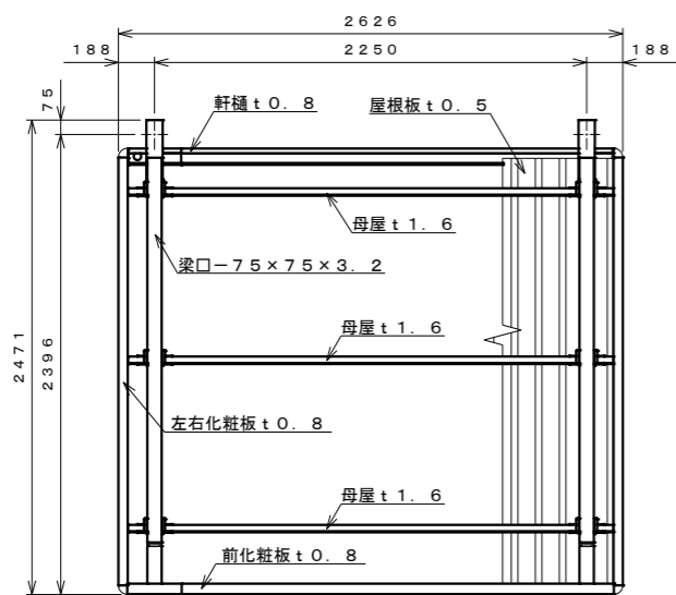
平面図 S=1:30
