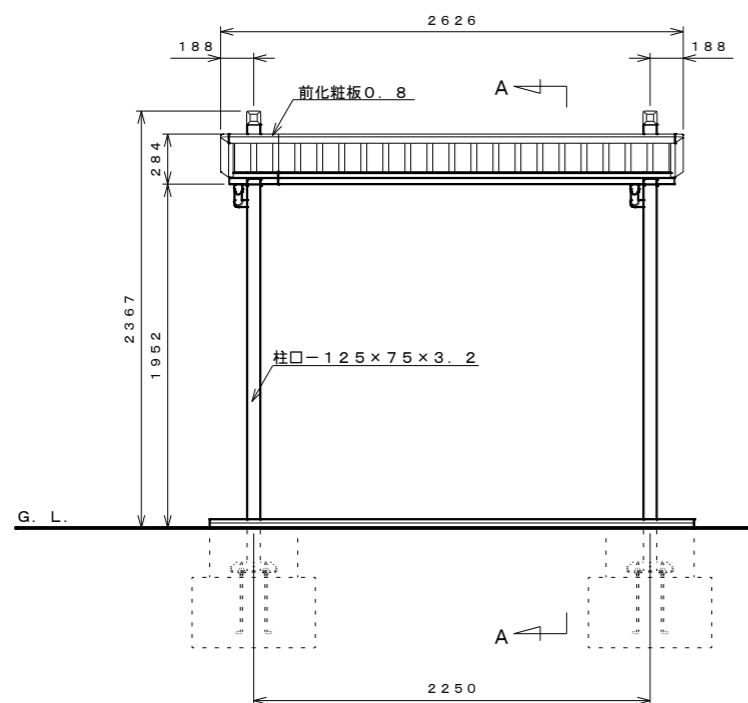
正面図 S=1:30
