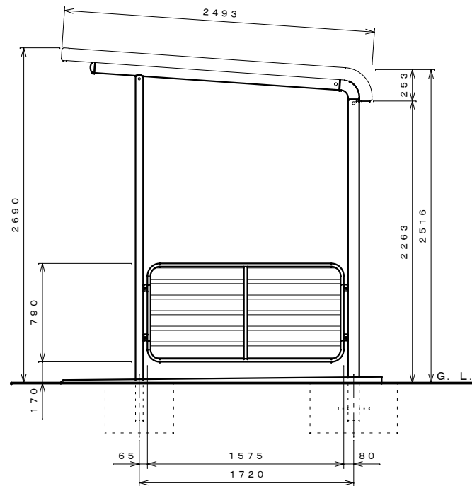
側面図 S=1:30
