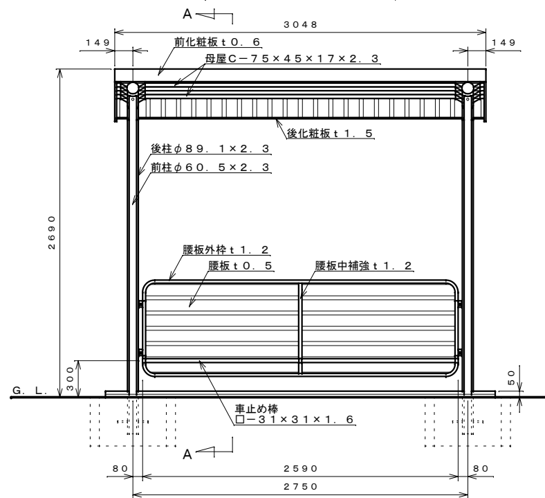
正面図 S=1:30
