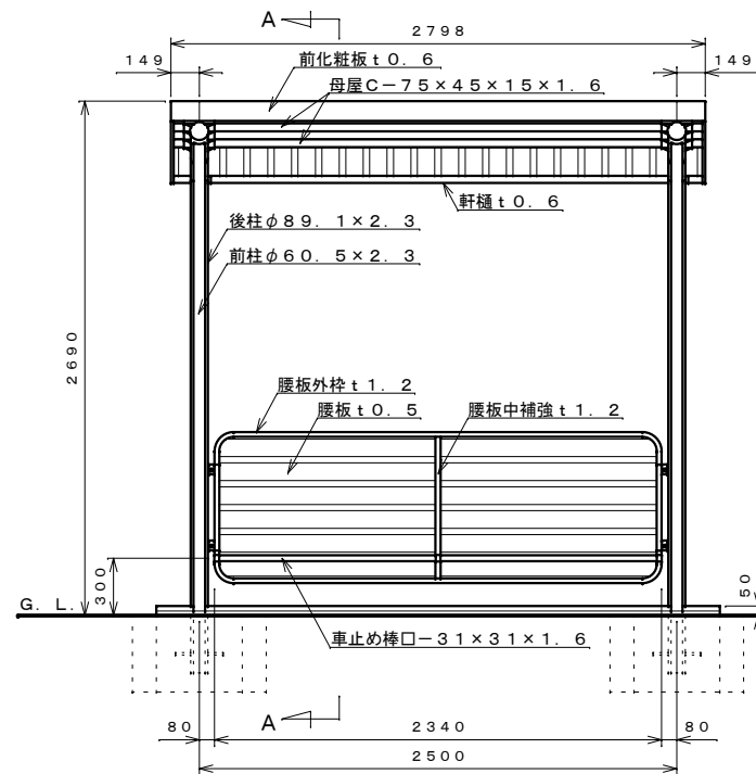
正面図 S=1:30
