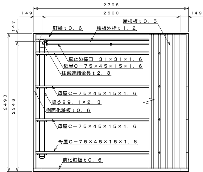
平面図 S=1:30
