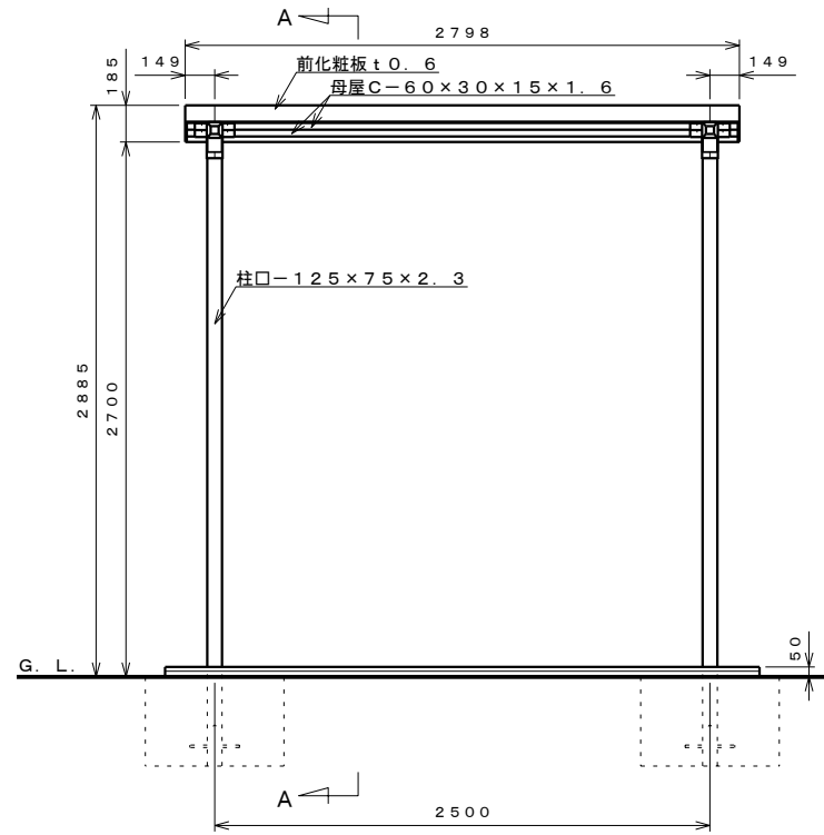
正面図 S=1:30
