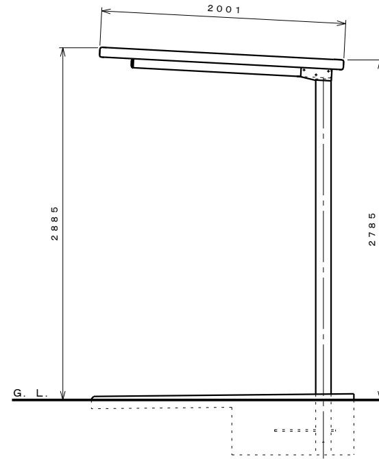
側面図 S=1:30
