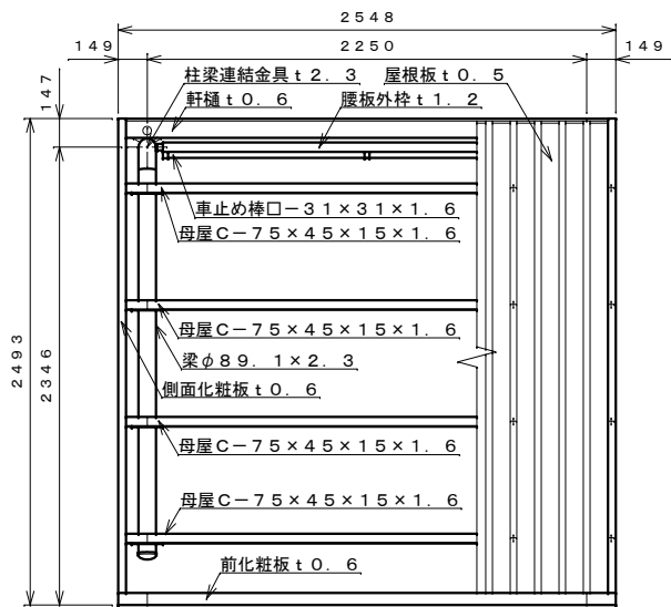
平面図 S=1:30
