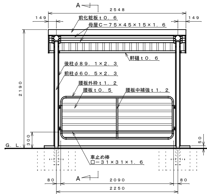
正面図 S=1:30
