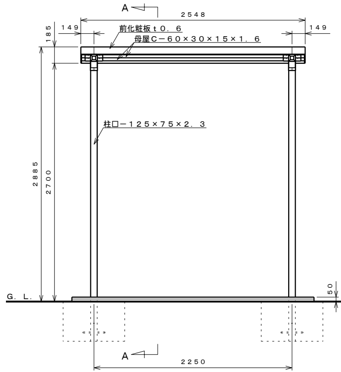
正面図 S=1:30
