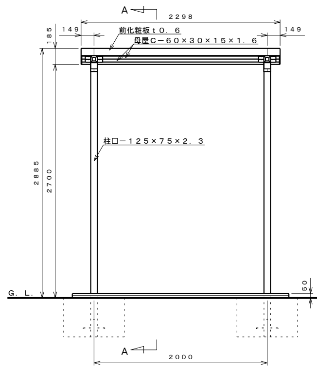
正面図 S=1:30
