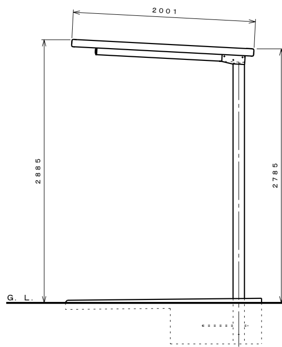
側面図 S=1:30
