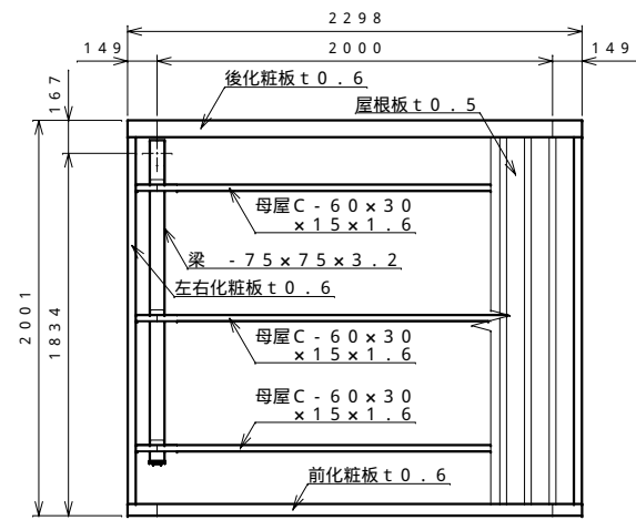
平面図 S = 1 : 30
