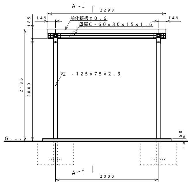
正面図 S = 1 : 30
