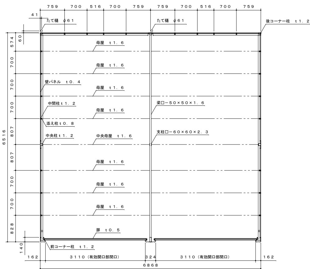
平面図 S=1:50
