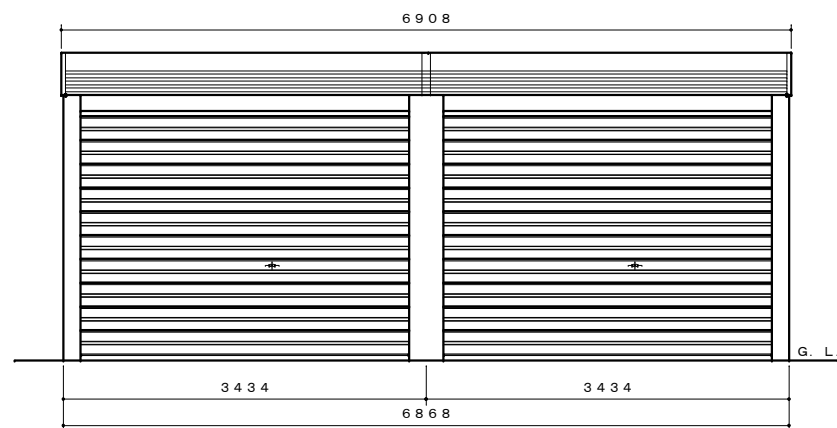
正面図 S=1:50
