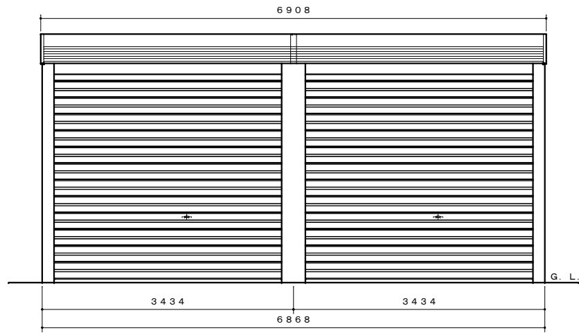
正面図 S=1:50
