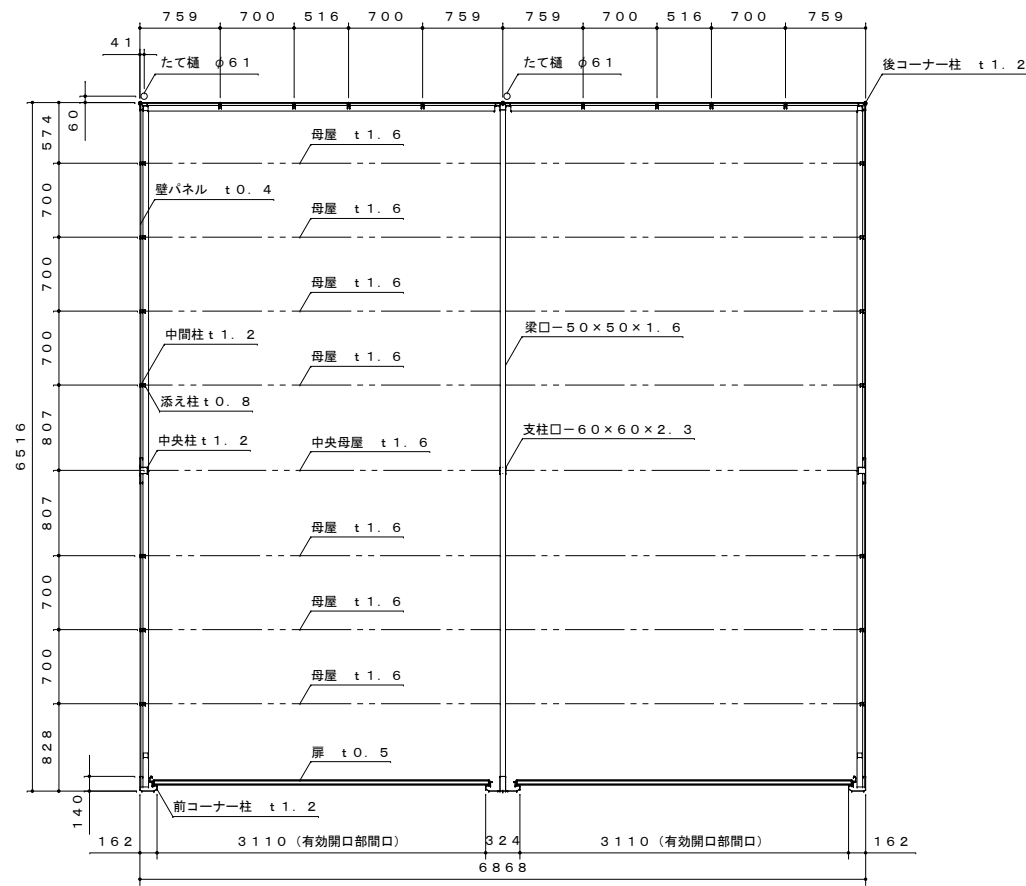
平面図 S=1:50
