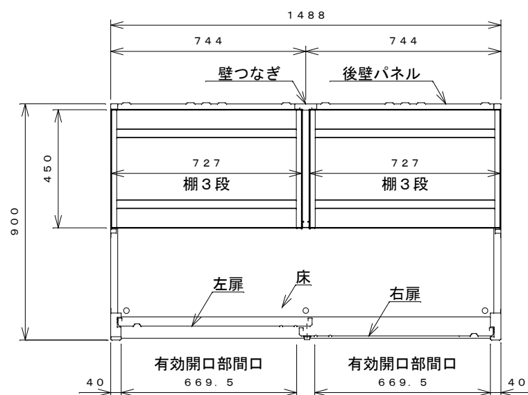
平面断面図
