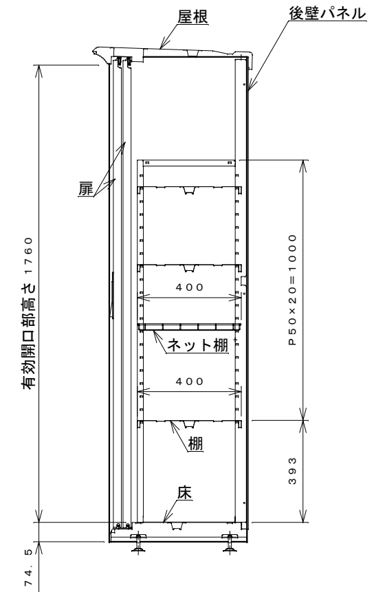
側面断面図
