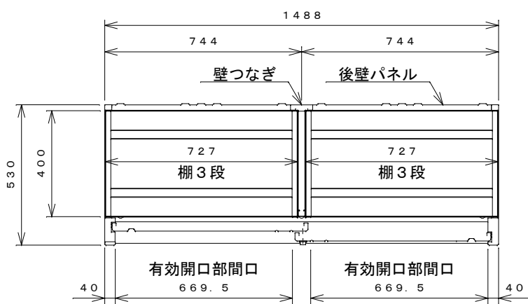
平面断面図
