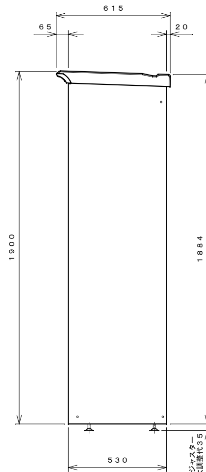
右側面図
