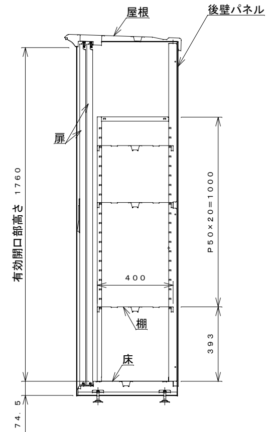
側面断面図
