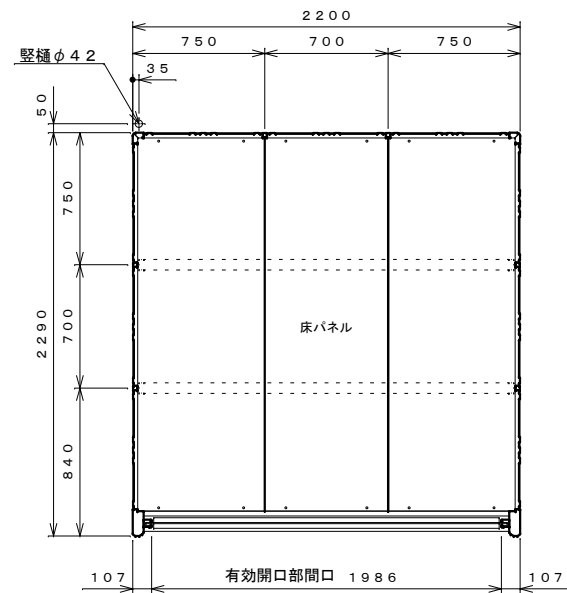
平面図 S=1:30
