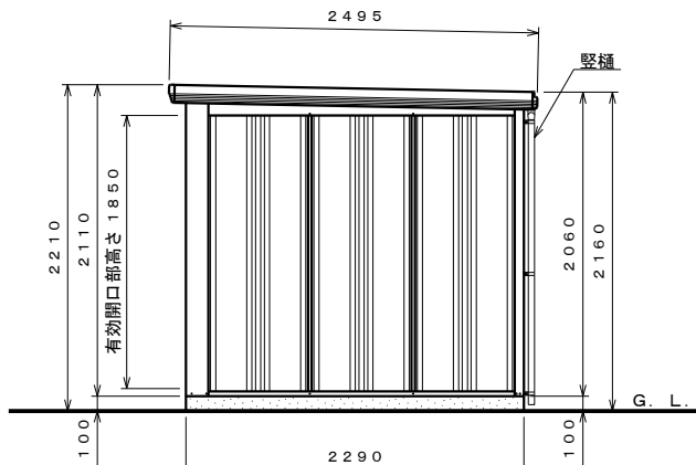
側面図 S=1:40
