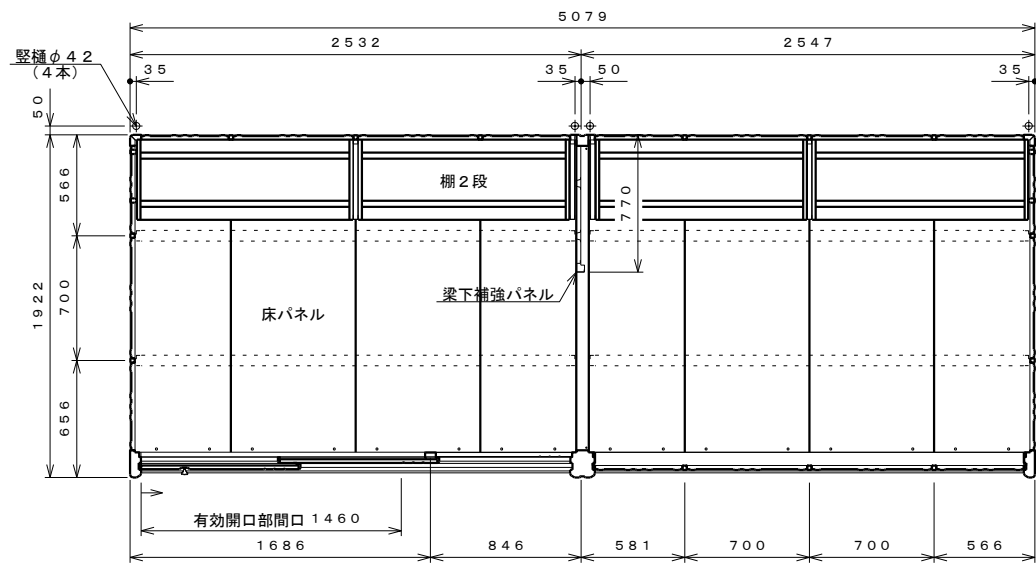
平面図 S=1:30
