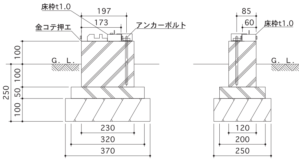
A-A断面図
