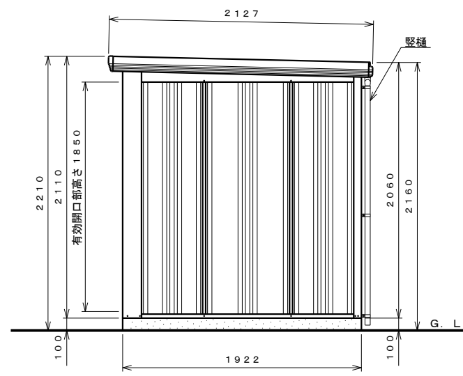
側面図 S=1:30
