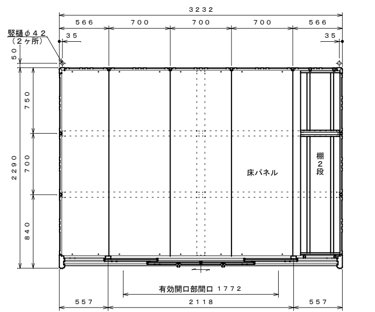
平面図 S=1:30
