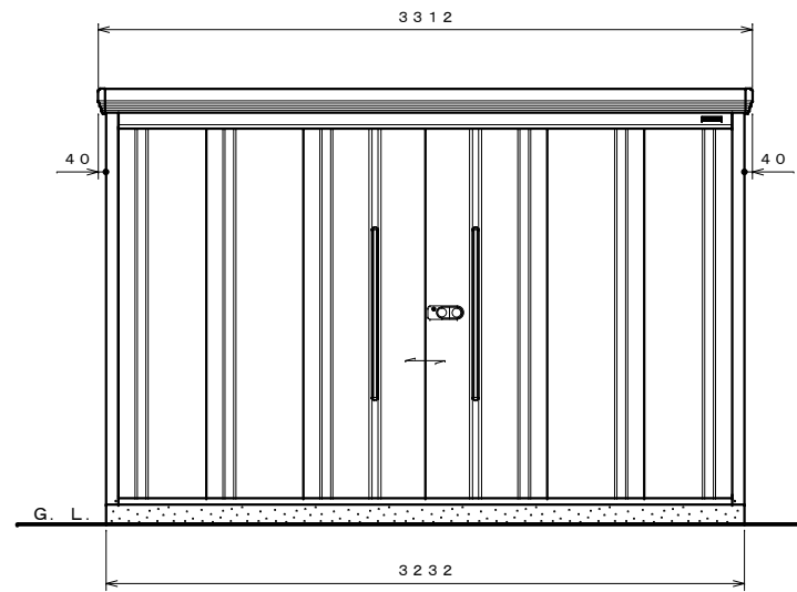
正面図 S=1:30
