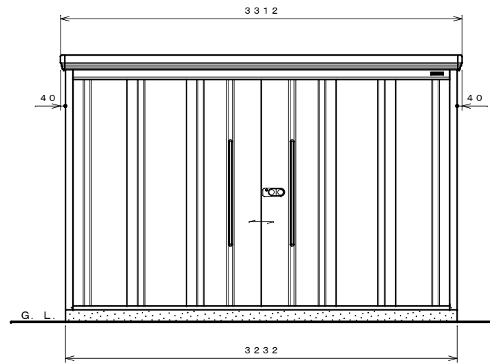
正面図 S=1:30
