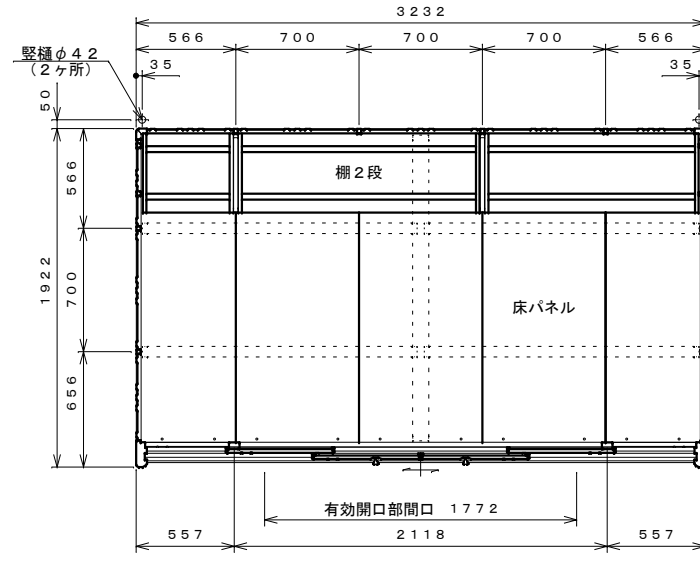
平面図 S=1:30
