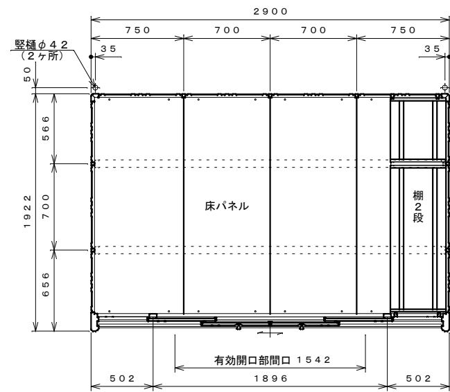
平面図 S=1:30
