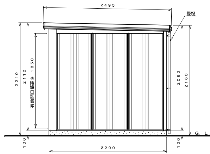
側面図 S=1:30
