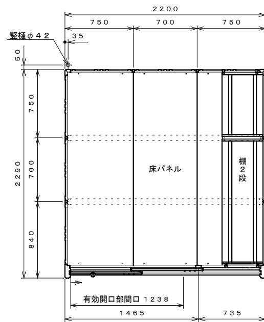
平面図 S=1:30
