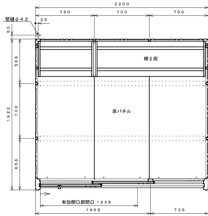
平面図 S=1:20
