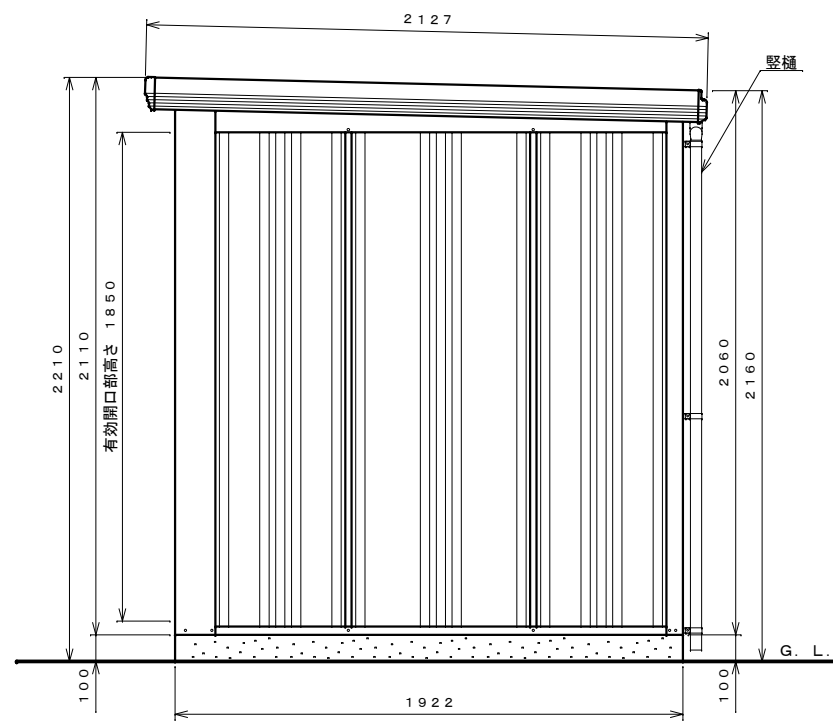
側面図 S=1:20
