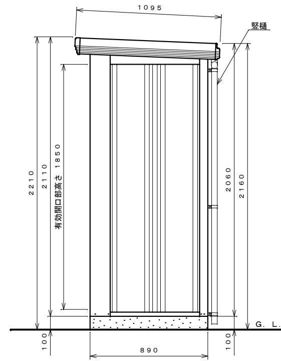
側面図 S=1:20
