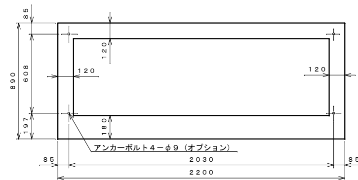
基礎伏せ図 S=1:20
