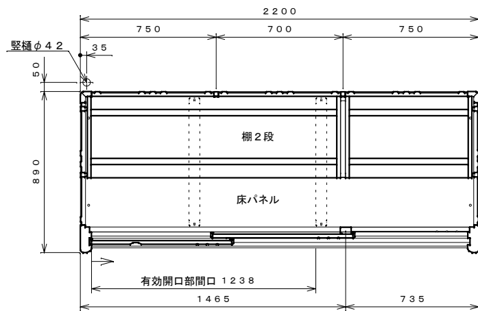
平面図 S=1:20
