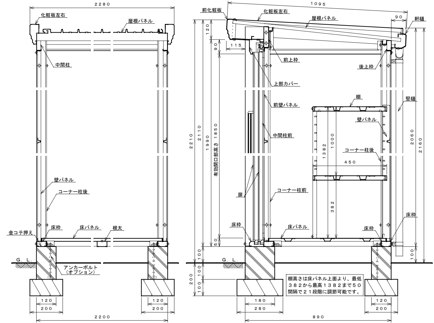
正面断面図 S=1:10
