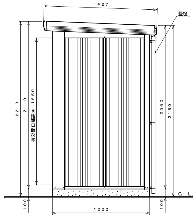
側面図 S=1:20
