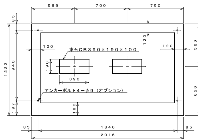
基礎伏せ図 S=1:20
