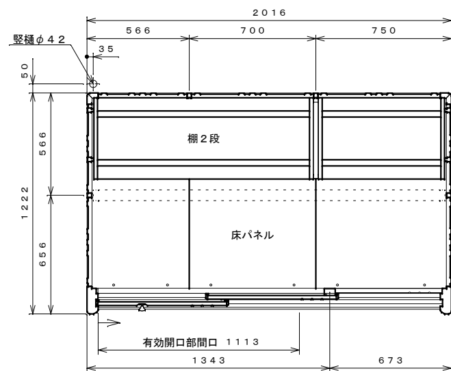
平面図 S=1:20
