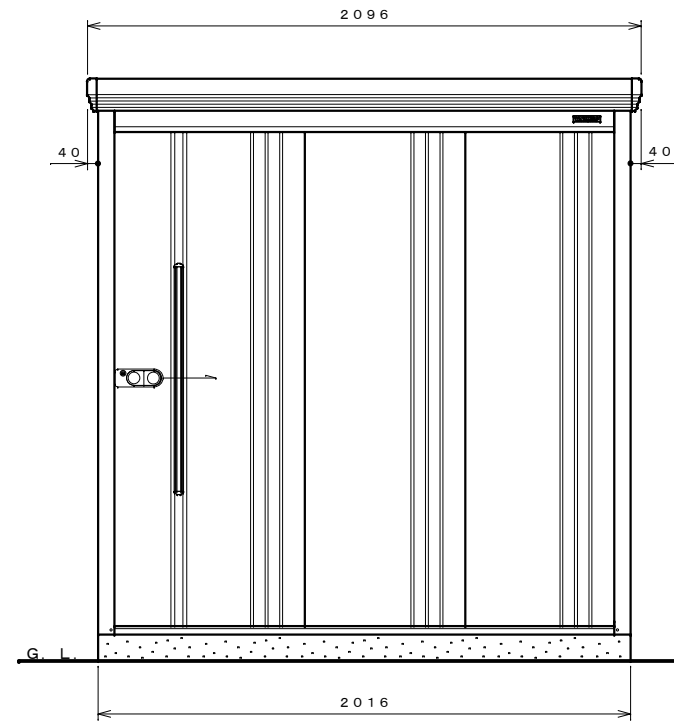
正面図 S=1:20
