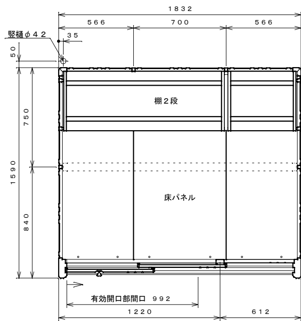
平面図 S=1:20
