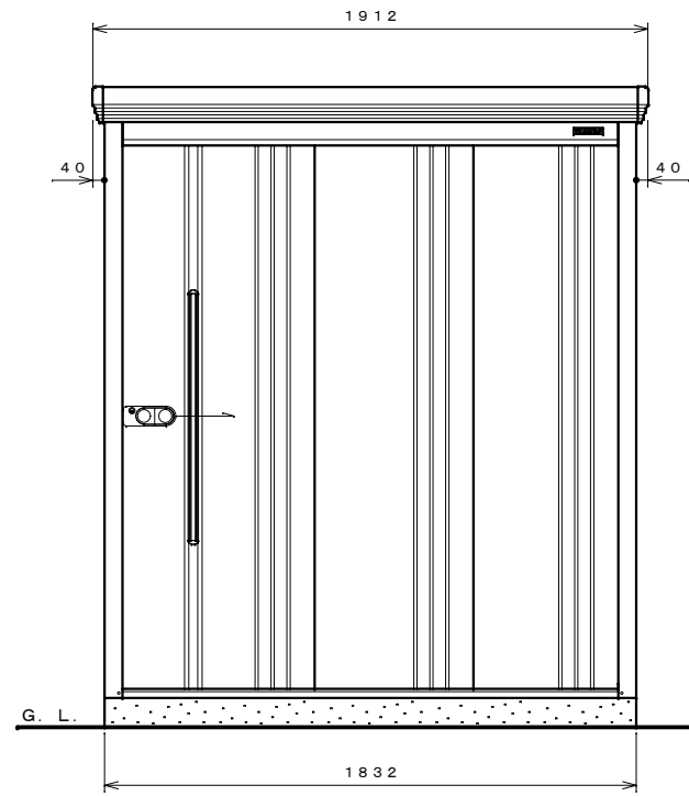
正面図 S=1:20
