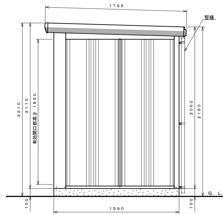
側面図 S=1:20
