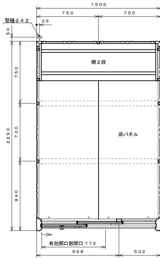
平面図 S=1:20
