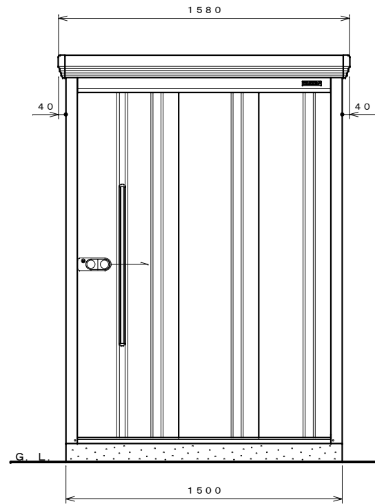
正面図 S=1:20
