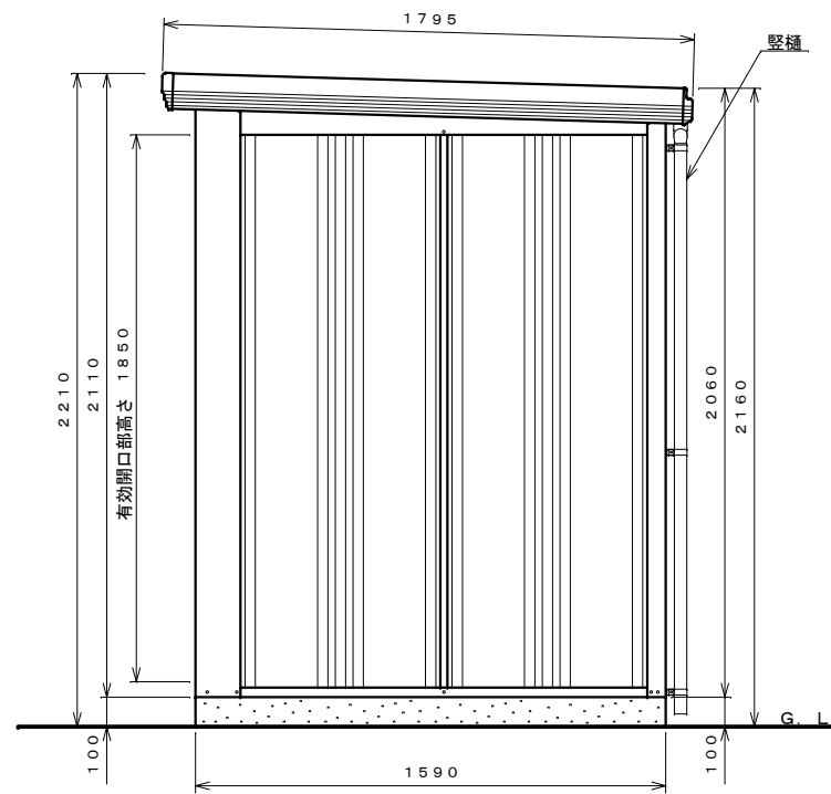
側面図 S=1:20
