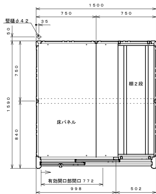
平面図 S=1:20
