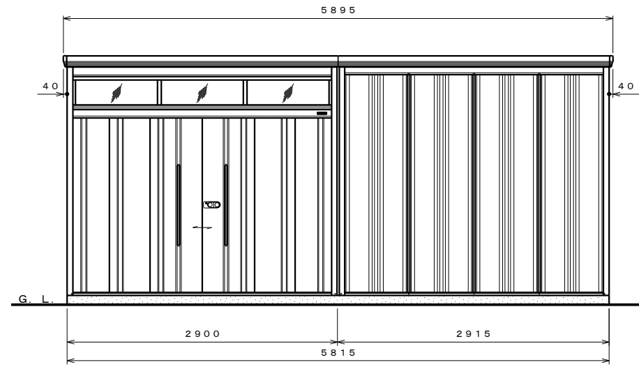
正面図 S=1:40
